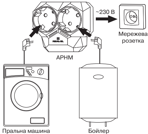
Мал. 2. Приблизна схема підключення
